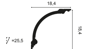
C338B BA'ROCK 200 x 18,4 x 18,4 cm Purotouch ®
