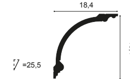
C338A BA'ROCK 200 x 18,4 x 18,4 cm Purotouch ®
